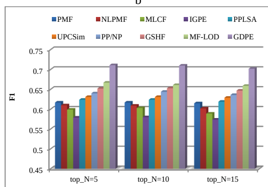
(شکل - ۴) مقایسه عملکرد در مجموعه داده Movielens 100K برحسب مقادیر مختلف top\_N : (a) معیار دقت، (b) معیار یادآوری، و (c) معیار F1 . سطح پراکندگی روی \theta=20\% تنظیم شده است.
