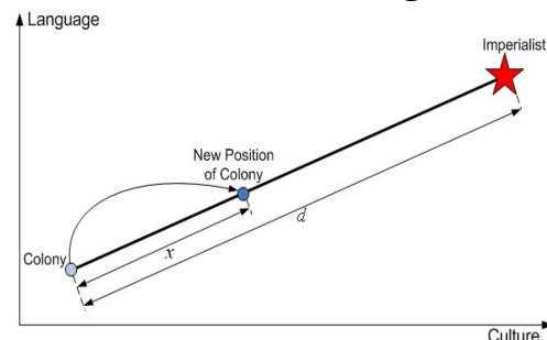
(شکل-۳): شمای کلی حرکت مستعمرات به سمت امپراتوری [۶] (Figure-3): Movement of colonies toward their relevant imperialist [6]
