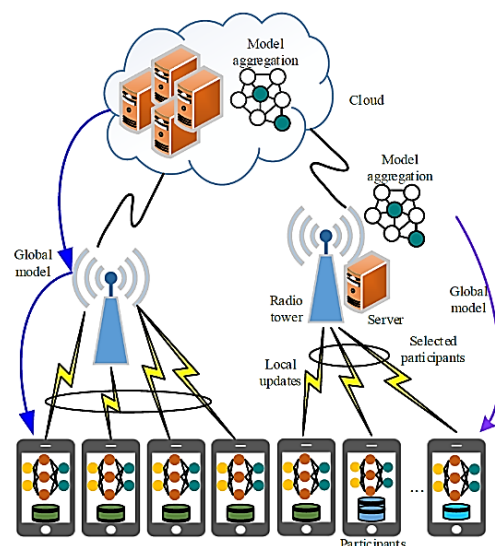
(شکل ۱۰-۱): نمای کلی FL در سامانه‌های اینترنت اشیا [۴۲]
