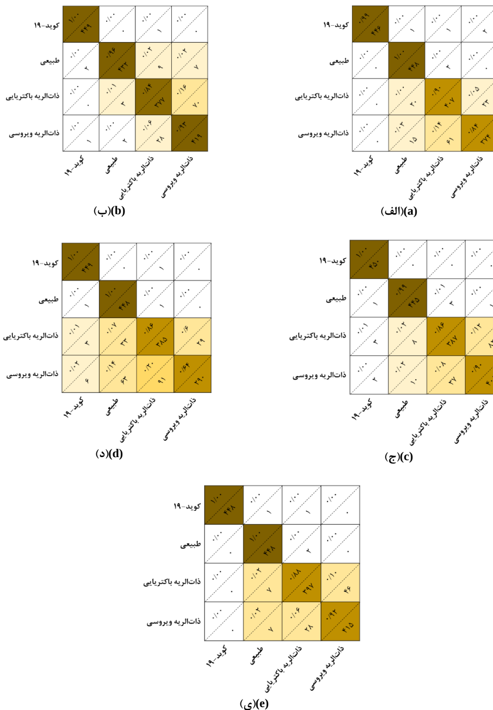
(شکل-۷): ماتریس درهم‌ریختگی نتایج با پنج مدل: (الف) مدل ۱، (ب) مدل ۲، (ج) مدل ۳، (د) مدل ۴، و (ی) مدل ۵
