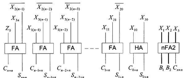
(شکل-۶): محاسبه B_1 و B_2 در مبدل معکوس [12] (Figure-6): B_1 and B_2 computations in reverse conversion [12]
