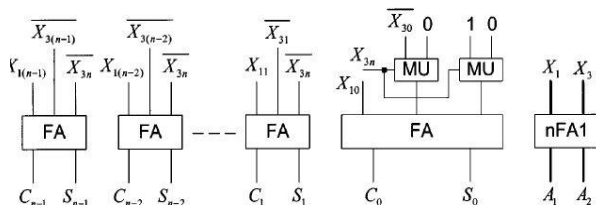
(شکل-۵): محاسبه A_1 و A_2 در مبدل معکوس [12] (Figure-5): A_1 and A_2 computations in reverse conversion [12]
