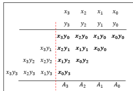
(شکل-۱۰): نحوه قرارگیری حاصل ضربهای جزئی
