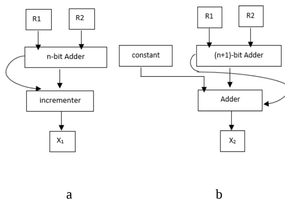
(شکل-۷): نمودار جعبه‌ای جمع کننده مانده‌ای در پیمانه (a) 2^n - 1 و (b) 2^n + 1
