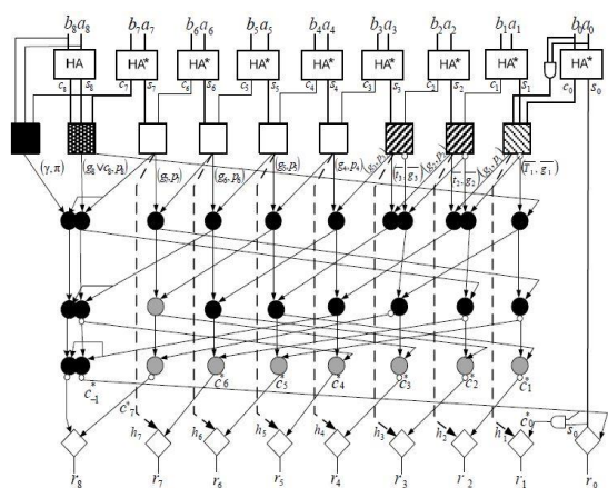
(شکل-۹): جمع کننده پیشوندی موازی در پیمانه 2^n + 1 [16] (Figure-9): Parallel prefix adder in modulo- 2^n + 1 [16]
