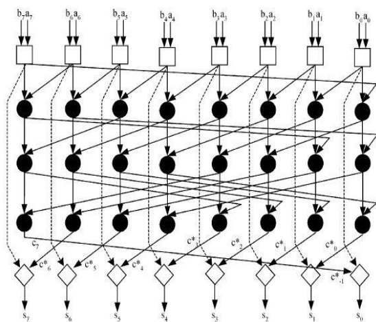
(شکل-۸): جمع کننده پیشوندی موازی در پیمانه 2^n - 1 [14] (Figure-8): Parallel prefix adder in modulo- 2^n - 1 [14]
