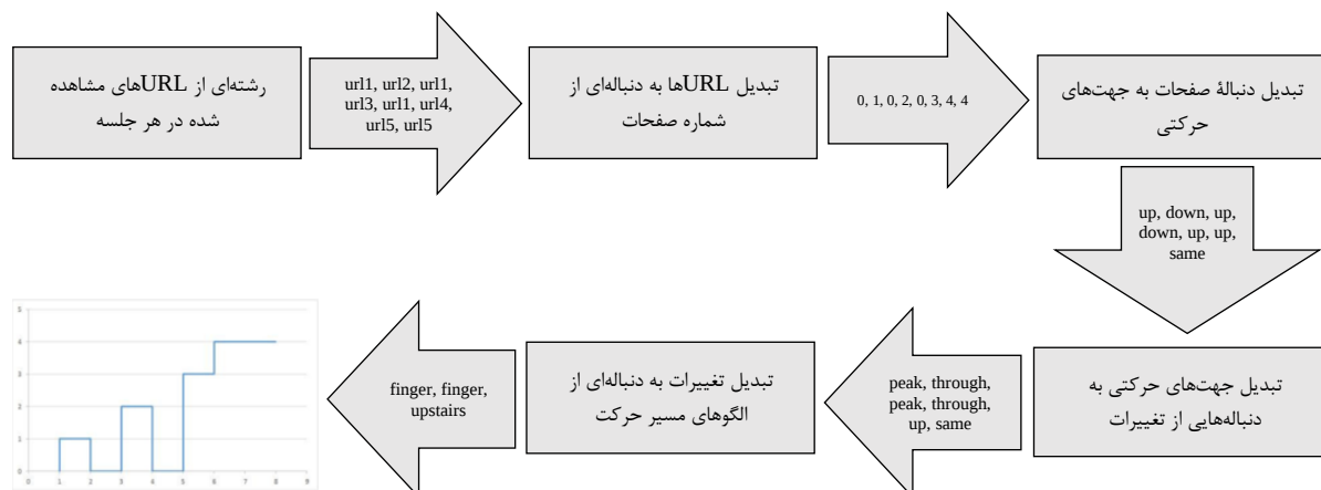
(شکل-۷): روش کشف خودکار الگو (APD) برای تبدیل یک توالی صفحه به نمودار گراف ردپا [رشته رفتار] (Figure-7): Automatic Pattern Discovery (APD) method for converting a page sequence into a footprint graph [behavior thread]
