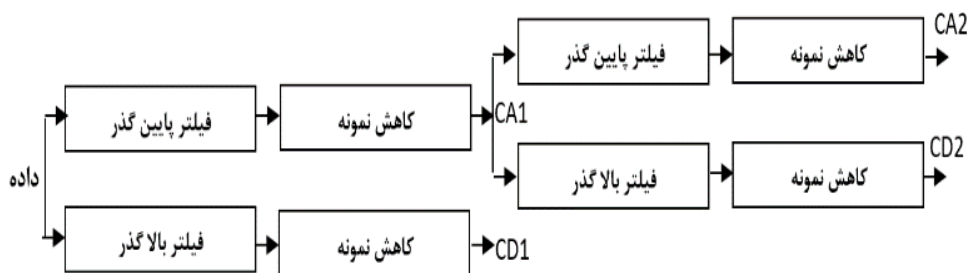
(شکل-۴): الگوریتم تبدیل موجک گسسته، ضرایب تقریب CAs و ضرایب جزئیات CDs (Figure-4): Discrete wavelet transform, CAs approximation coefficients and CDs detail coefficients
