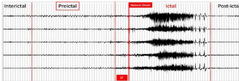
(شکل-۱): نمونه‌ای از پنج کانال نوار مغزی صرعی [3] (Figure-1): An example of five epileptic EEG channels [3]
