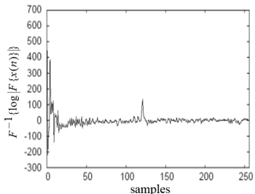
(شکل-۸): معکوس تبدیل فوریه گسسته، لگاریتم، تبدیل
