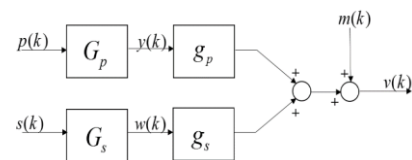
(شکل ۱۰): مدل غیرایستادن و غیرخطی نوار مغزی صرعی
