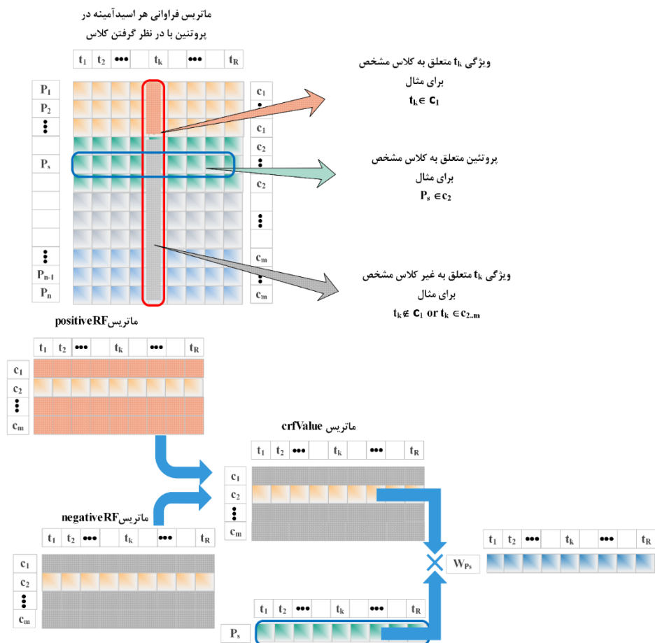
(شکل - ۱) مراحل روش استخراج ویژگی با استفاده از روش TFCRF (Figure- 1) The steps of the feature extraction method using the TFCRF method
