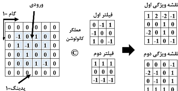
(شکل-۳): عملکرد لایه کانولوشن در شبکه کانولوشنال (Figure-3): The function of convolution layer in CNN network
