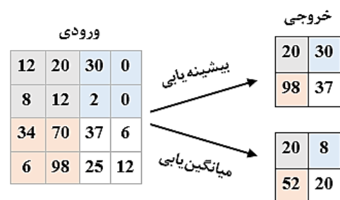
(شکل-۶): مقایسه عملکرد لایه نمونه بردار کاهنده در دو حالت میانگین یابی و بیشینه یابی (گام = ۲؛ پدینگ = ۰؛ ابعاد پنجره = ۲×۲)
