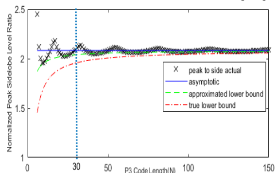
(شکل-۵): نسبت PSLR کد P3 نرمالیزه شده با ریشه طول کد N. در شکل علامت × بیان‌گر نسبت دقیق، - مقدار مجانبی، -- کران پایین تقریب زده شده و - کران پایین واقعی است. (Figure-5): PSLR for P3 Normalized by the square root of the sequence code length N. In the plot, × indicates the exact ratio, - the asymptotic value, -- the approximated lower bound and - true lower bound.
