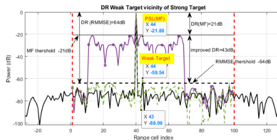
(شکل-۶): مقایسه گستره پویایی الگوریتم RMMSE
