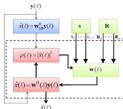
(شکل ۳): نمودار گردشی الگوریتم FFL-APCR [7] (Figure-3): Flowchart of FFL-APCR algorithm
