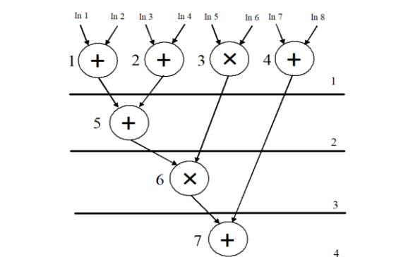
(شکل-۴): نمونه‌ای از DFG زمان‌بندی شده شکل (۲)
