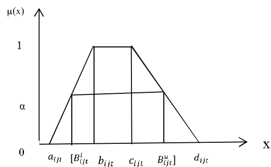
(شکل ۱-): تابع عضویت دوزنقه‌ای و برش-α [24] (Figure-1): Trapezoidal membership function and α-cut [24]
