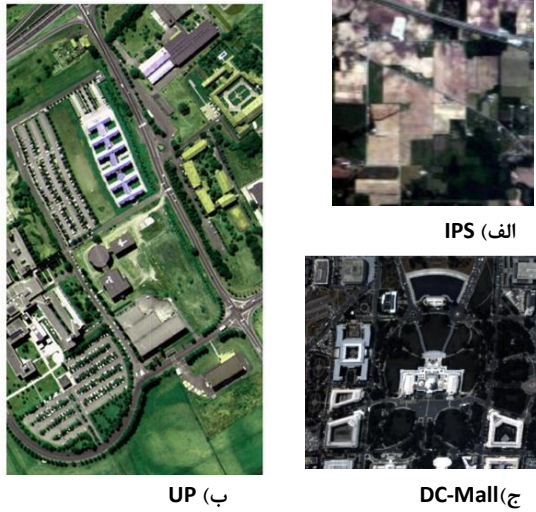
(شکل ۲- (الف) تصویر با رنگ کاذب ایندیانا (ب) تصویر با رنگ کاذب دانشگاه پاوایا (ج) تصویر با رنگ کاذب DC-Mall (Figure 2) The Original Data of (a) IPS, (b) UP, (c) DC-Mall
