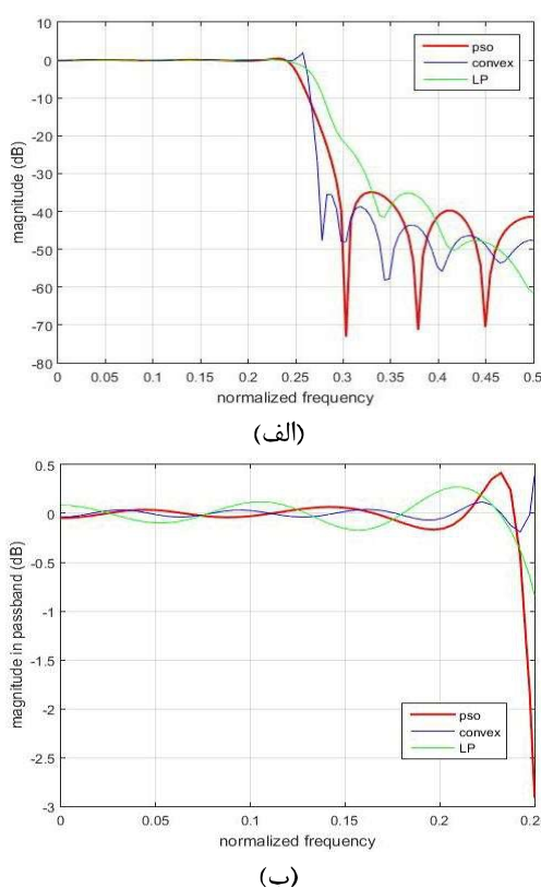
(شکل-۷): پاسخ اندازه فیلتر پایین گذر طراحی شده با روش بهینه‌سازی PSO و برنامه‌ریزی محدب و برنامه‌ریزی خطی. (Figure-7): Magnitude of designed lowpass filters in passband by PSO, convex, and LP methods.
