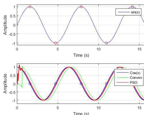
(شکل-۱۲): سیگنال سینوس و مشتق آن با دو مشتق‌گیر
