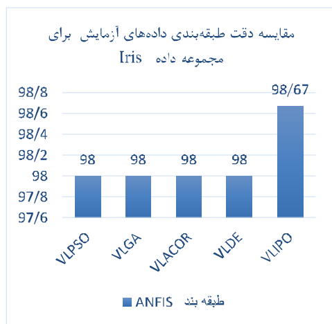
(نمودار-۲): مقایسه دقت طبقه‌بندی داده آزمایش برای مجموعه داده Iris در طبقه‌بند ANFIS از طریق روش‌های ابتکاری با طول متغیر (Diagram-2): Comparing accuracy of test data classification for Iris dataset in ANFIS class through innovative methods with various lengths
