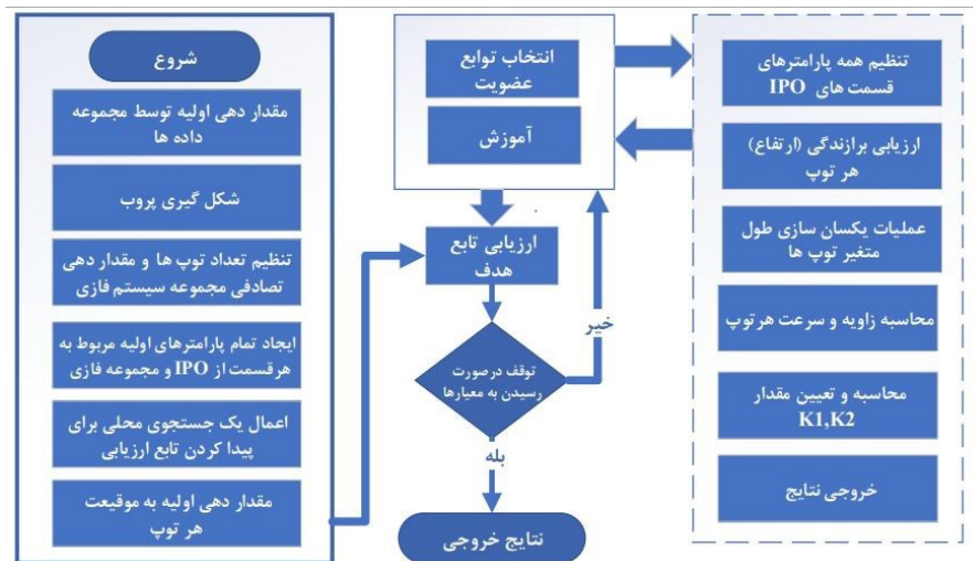
(شکل-۱۰): روندنمای کلی فرآیند روش پیشنهادی توسط روش VLIPPO (Figure-10): Overall flowchart of proposed method's process via VLIPPO method
