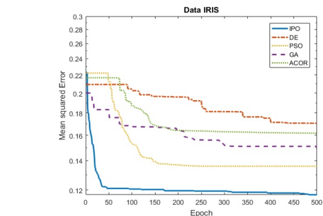
(شکل-۱۶): هم‌گرایی مقدار MSE برای مجموعه‌داده Iris برای طبقه‌بند ساده ANFIS (Figure-16): Convergence of MSE value for Iris data set for simple ANFIS classifier
