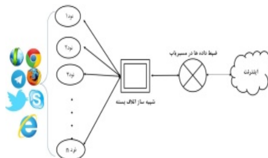
(شکل-۱): معماری سامانه جهت شبیه‌سازی رخداد اتلاف بسته و ضبط داده‌ها (Figure-1): System Structure to Emulate Packet Loss and Data Capturing
