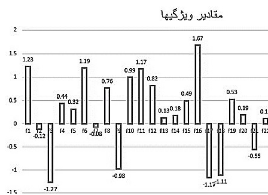
(شکل-۴): ضرایب توان معادله رگرسیون غیرخطی
