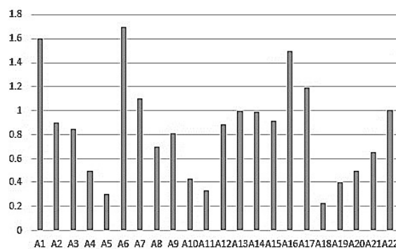
(شکل-۵): ضرایب تأثیر هر ویژگی مربوط به رگرسیون
