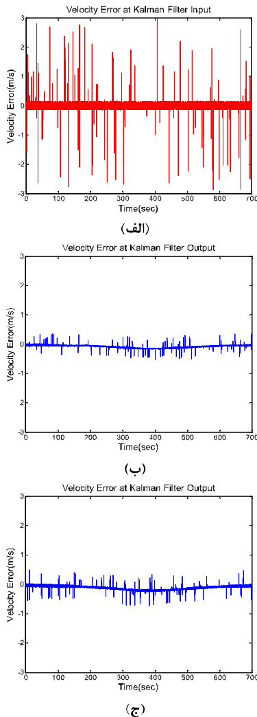
(شکل-۵). نمودار خطای تخمین سرعت هدف (الف) بدون فیلتر کالمن (ب) با اعمال فیلتر کالمن در نرم‌افزار (ج) با اعمال فیلتر کالمن در سخت‌افزار.
