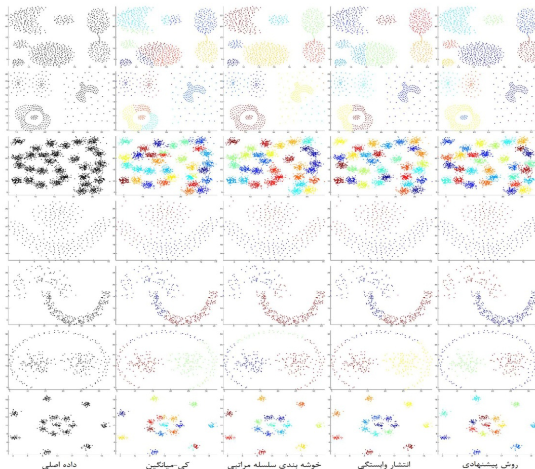
(شکل-۲): شبیه‌سازی‌ها بر روی هفت شکل متفاوت. هر سطر روش پیشنهادی را با دیگر روش‌های موجود و پرکاربرد مقایسه می‌کند. شکل‌های مختلف شامل تعداد متفاوتی خوشه هستند.
