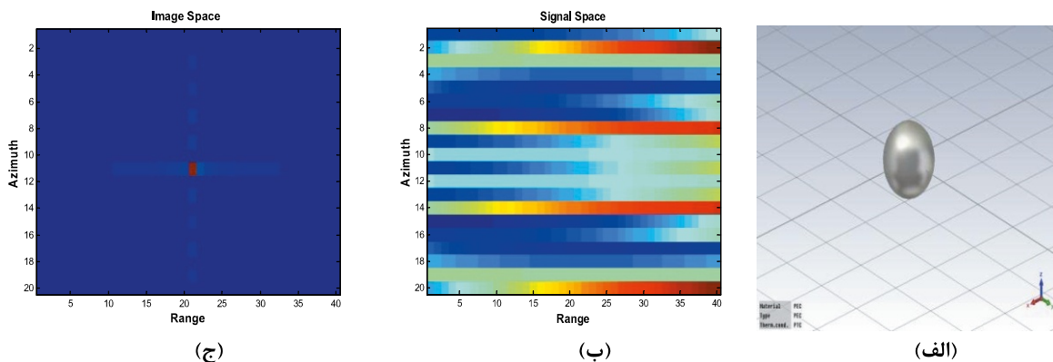
(شکل-۱۳): الف) جمع‌آوری داده‌های خام در محیط نرم‌افزاری CST. ب) انتقال داده‌های خام از CST به MATLAB و تشکیل فضای سیگنالی. (Figure-13): a) Raw data acquisition in CST software environment. b) Transferring of raw data from CST to MATLAB and signal space formation. c) Applying the PFA algorithm on the signal space and image space formation.
