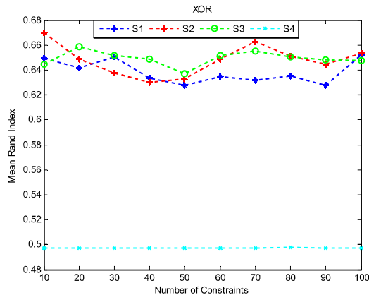
(شکل-۴): متوسط RI روش‌های مختلف بر روی داده XOR. به‌ازای تعداد قیدهای متفاوت. S1 ساختار یک، S2 ساختار دو، S3 ساختار سه، S4 ساختار چهار
