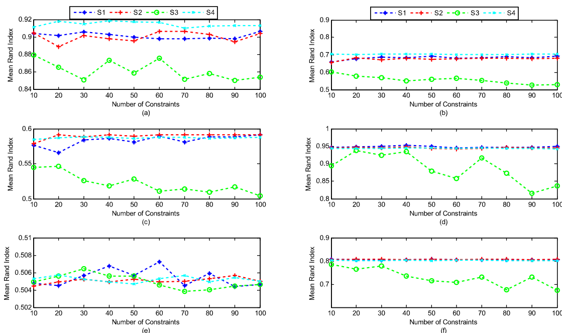
(شکل-۶): متوسط RI روش‌های مختلف بر روی داده UCI. به ازای تعداد قیدهای متفاوت. (S1) ساختار یک، (S2) ساختار دو، (S3) ساختار سه، (S4) ساختار چهار. Soybean (a)، Heart (b)، Ionosphere (c)، Wine (d)، Sonar (e)، Iris (f).
