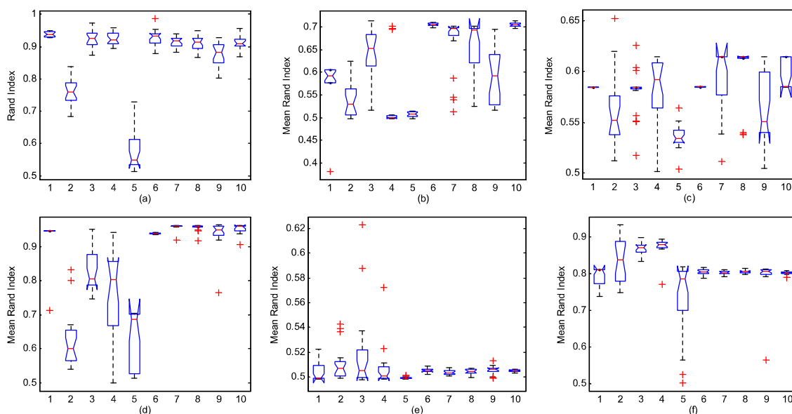
(شکل-۵): نتایج خوشه‌بندی الگوریتم‌های مختلف بر روی داده‌های پایگاه داده UCI. (۱) فاصله اقلیدسی، (۲) RCA [17]، (۳) Xiang [11]، (۴) kernel- \beta [20]، (۵) unweighted-S [26]، (۶) DMKL [27]، (۷) ساختار یک، (۸) ساختار دو، (۹) ساختار سه، (۱۰) ساختار چهار. Soybean (a)، Heart (b)، Ionosphere (c)، Wine (d)، Sonar (e)، Iris (f).
