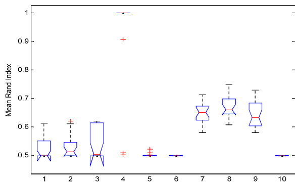
(شکل-۳): نتایج خوشه‌بندی الگوریتم‌های مختلف بر روی داده XOR (۱. فاصله اقلیدسی، ۲. RCA [17]، ۳. Xiang [11]، ۴. kernel- \beta [20]، ۵. unweighted-S [26]، ۶. DMKL [27]، ۷. ساختار یک، ۸. ساختار دو، ۹. ساختار سه، ۱۰. ساختار چهار) (Figure-3): Clustering results of different algorithms for XOR dataset. 1) Euclidean, 2) RCA [17], 3) Xiang [11], 4) kernel- \beta [20], 5) unweighted-S [26], 6) DMKL [27], 7) structure 1, 8) structure 2, 9) structure 3, 10) structure 4
