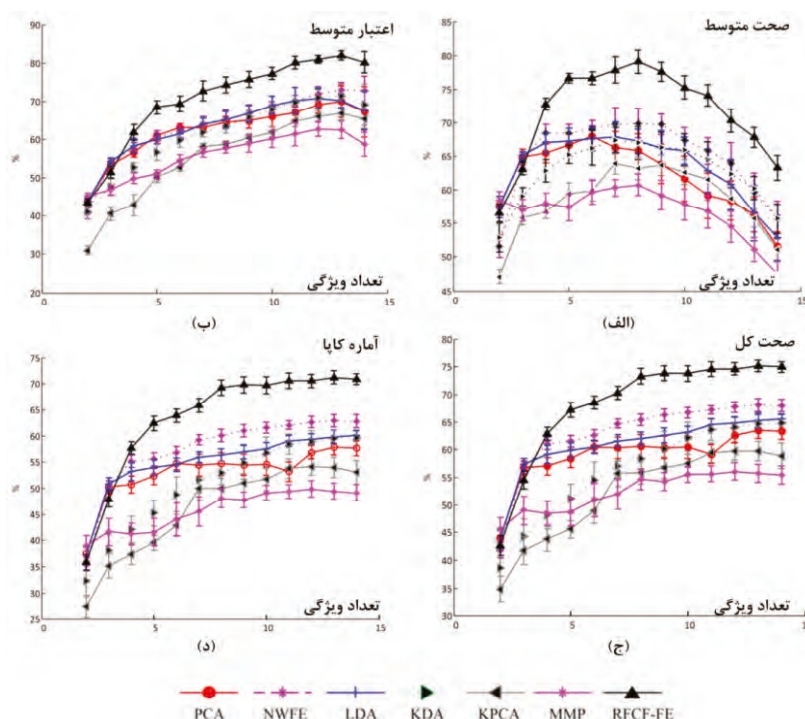
(شکل - ۳): معیارهای ارزیابی طبقه‌بندی برای تصویر IPS به ازای روش‌های مختلف استخراج ویژگی و تعداد متفاوت ویژگی‌ها (الف) صحت متوسط (ب) اعتبار متوسط (ج) صحت کل (د) آماره کاپا (Figure- 3): Classification accuracy measures for IPS data set using different FE methods and various numbers of features, (a) Average accuracy (b) Average validity (c) Overall accuracy (d) Kappa statistic
