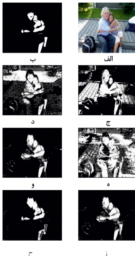
(شکل ۷- الف: تصویر اصلی، ب: Ground truth، نقشه احتمال پوست برای ویژگی‌های جداساز معرفی شده: (ج-ه) هم‌اتفاقی خودی R، |R-G| و max(R,G,B)-min(R,G,B)، (و-ح) هم‌اتفاقی متقابل R&A، R&Y و R&B (Figure-7): from top/right to down/left: Input image, Ground Truth, Skin probability maps based on self/cross co-occurrence discriminant features such as R, |R-G|, max(R, G, B)-min(R, G, B), R&A, R&Y and B&M.
