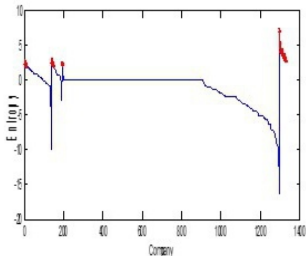
(شکل-۳): تابع آنترپی سهام (Figure-3): stock entropy function
