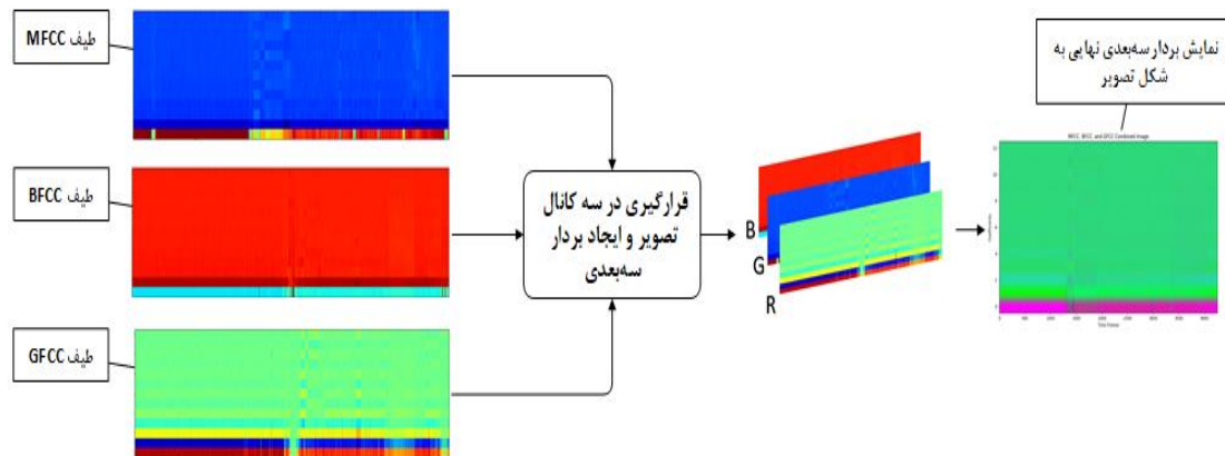
و ایجاد یک بردار سه بعدی GFCC و BFCC و MFCC (شکل-۶): ترکیب سه طیف (Figure-7): Combining the three spectra MFCC, BFCC, and GFCC and creating a 3D vector vector
