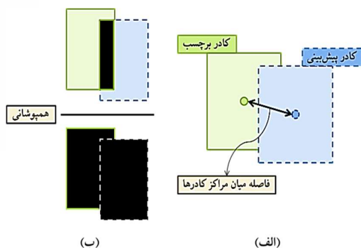
(شکل ۳): (الف) فاصله میان مراکز کادرهای برچسب و پیش‌بینی معیاری برای دقت ردیابی، (ب) هم‌پوشانی میان کادرها معیاری برای موفقیت ردیابی (Figure-3): (Right) Distance between the center of groundtruth and prediction bounding boxes as the tracking precision, (Left) Intersection over union as the tracking success
