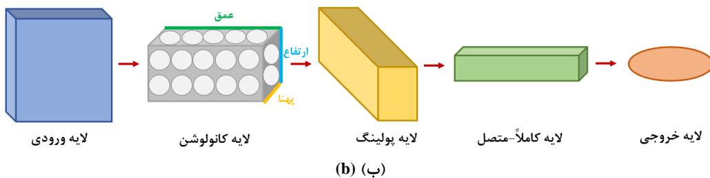
(شکل-۵): تفاوت شبکه‌های عصبی معمولی و شبکه عصبی کانولوشن. (الف) شبکه عصبی معمولی، و (ب) شبکه عصبی کانولوشن (Figure-5): Difference of conventional neural networks and convolutional neural networks. (a) Conventional neural networks, and (b) convolutional neural network
