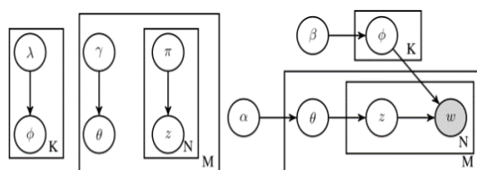
(ب) مدل LDA توسعه داده شده تقریبی (آ) مدل LDA توسعه داده شده
