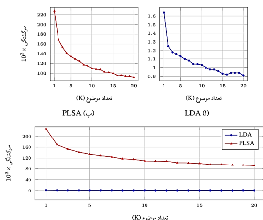
(ج) سرگشتگی LDA و PLSA در یک نمودار
