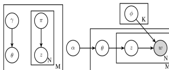
(ب) مدل گرافی تقریبی LDA (ا) مدل گرافی LDA (شکل-۲): الگوی گرافی LDA به همراه مدل ساده‌شده آن [۱۰].
