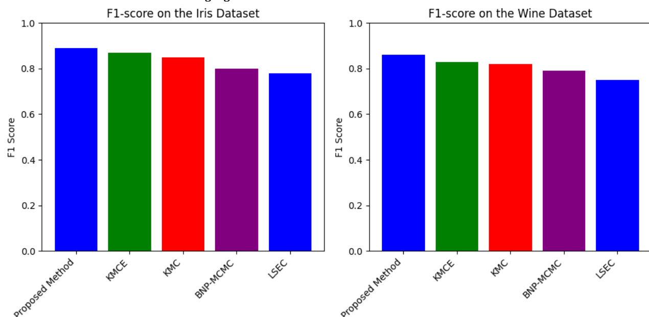
(شکل-۱۱): مقایسه نموداری امتیاز F1 برای روش پیشنهادی در مقابل روش‌های خوشه‌بندی KMCE, KMC, BNP-MCMC و LSEC بر روی دو مجموعه داده Iris و Wine
