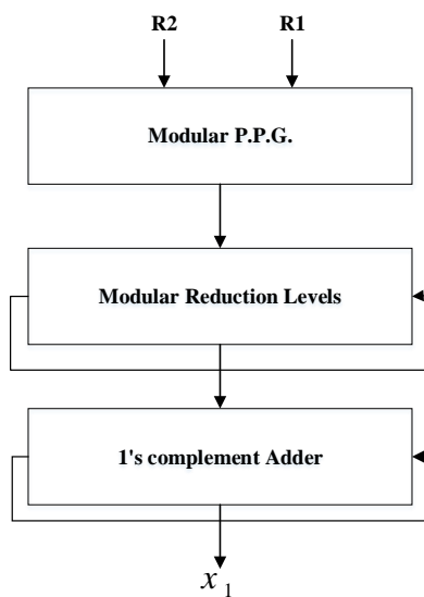
(شکل-۱۳): نمودار جعبه‌ای ضرب‌کننده در پیمانۀ 2^n - 1
