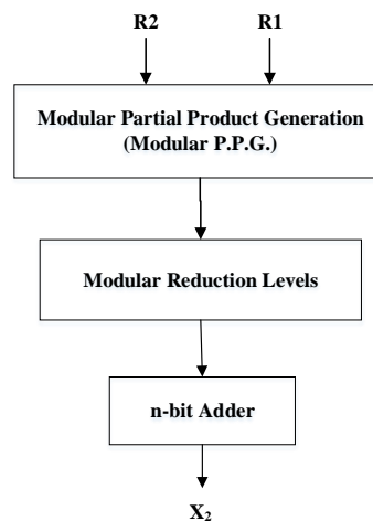
(شکل-۱۱): نمودار جعبه‌ای ضرب‌کننده در پیمانۀ 2^n
