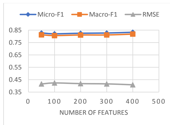
(شکل-۱۸): نتایج درخت تصمیم برای روش CC&DF (Figure-18): Decision Tree (DT) results for CC&DF method
