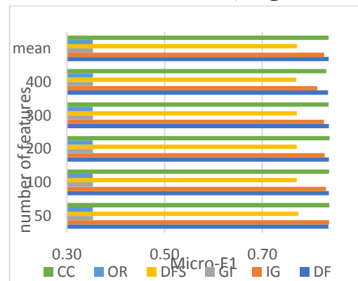
(شکل-۴): نتایج ماشین بردار پشتیبان برای روش‌های فردی (Figure-4): Support vector machine results for individual methods
