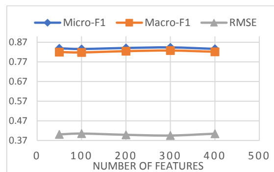
(شکل-۷): نتایج ماشین بردار پشتیبان برای روش CC&DF
