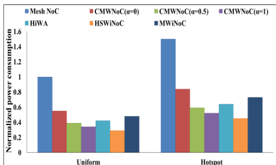
(شکل-۱۰): مقایسه میانگین توان مصرفی معماریهای مورد مطالعه تحت ترافیکهای Turbo-dec و RT-10x10 (Figure-10): Comparison of average power consumption of the considered architectures under Turbo-dec and RT-10x10 traffics.
