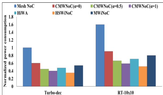
(شکل-۹): مقایسه میانگین توان مصرفی معماریهای مورد مطالعه تحت ترافیکهای یک نواخت و نقطه داغ (Figure-9): Comparison of average power consumption of the considered architectures under uniform and hotspot traffics.
