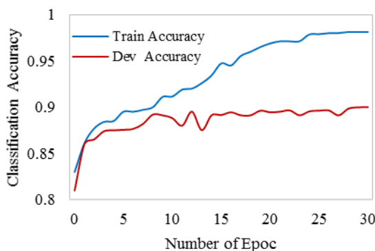
(شکل ۴-): ارزیابی مدل CNN-Attention-RNN-Plus-2channel. شکل سمت چپ دقت دسته‌بندی را برای نمونه‌های آموزشی و ارزیابی در ایپاک‌های مختلف شکل سمت راست میزان خطای کراس آنترینی را برای نمونه‌های آموزشی و ارزیابی در ایپاک‌های مختلف نشان می‌دهد.
