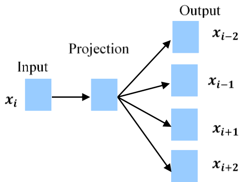
(شکل-۲): ساختار مدل اسکپ‌گرام [27] (Figure-2): Skip-Gram model structure [27]
