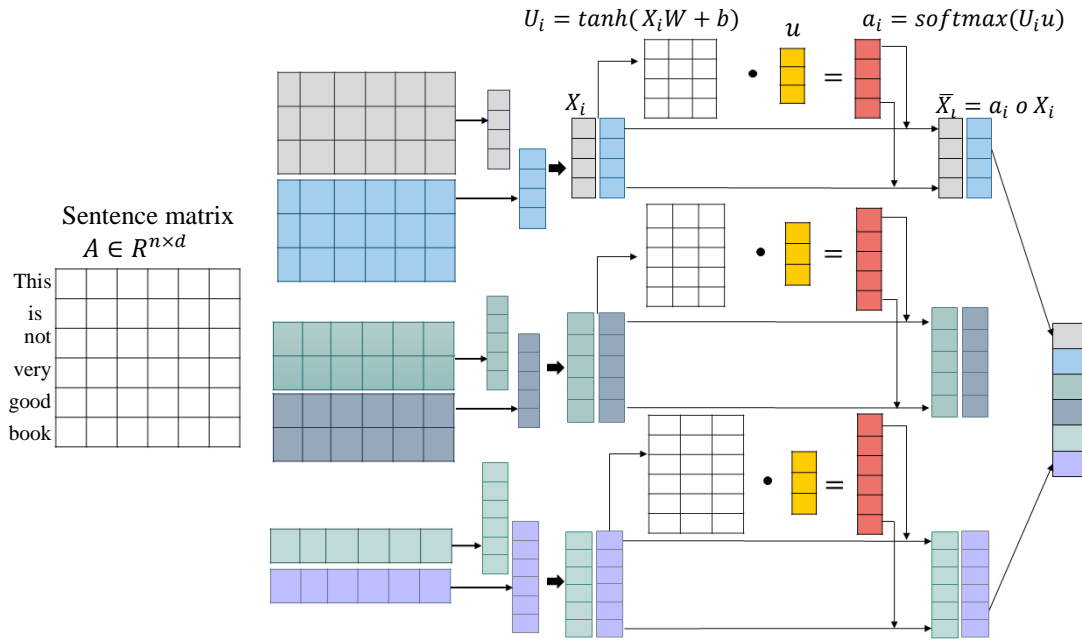
(شکل-۳): نمای کلی لایه پیچشی بر پایه سازوکار توجه (Figure 3): Overall Diagram of the convolutional layer based on attention mechanism
