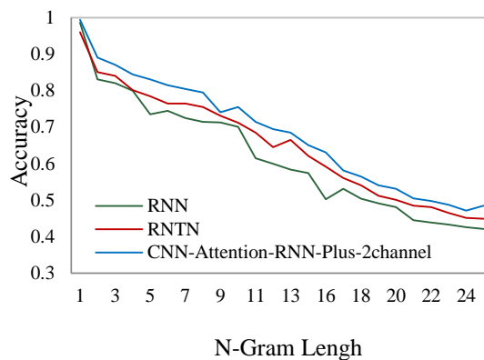
(شکل-۵): مقایسه دقت مدل‌ها بر اساس اندازه طول n-گرام (Figure-5): Comparison of the accuracy of various models based on n-gram length
