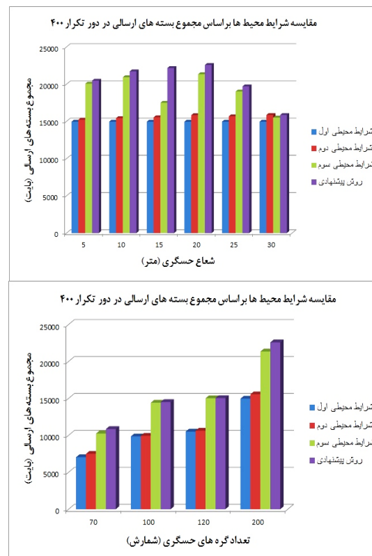
(شکل-۱۴): مقایسه روش‌ها بر اساس بازدهی شبکه
