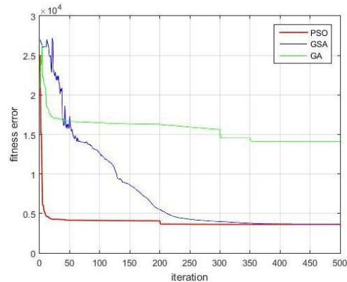
(شکل-۵): نمودار میزان خطای تابع هزینه بر حسب تعداد تکرارها برای سه الگوریتم PSO, GSA و GA. (Figure-5): Error vs. iterations for algorithms PSA, GSA, and GA.
