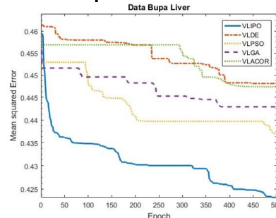
(شکل-۲۳): هم‌گرایی مقدار MSE برای مجموعه داده Bupa Liver برای طبقه‌بند ANFIS با روش‌های ابتکاری با طول متغیر
