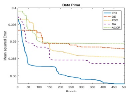
(شکل-۲۴): هم‌گرایی مقدار MSE برای مجموعه داده Pima Liver برای طبقه‌بند ساده ANFIS
