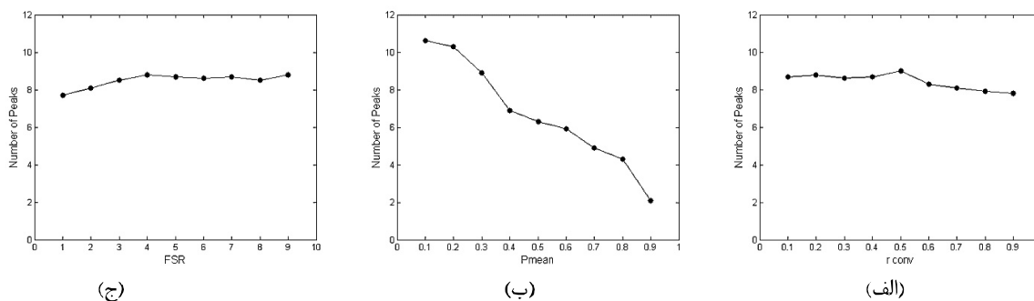
(شکل-۲): (الف) تأثیر تغییر r_{conv} بر تعداد قله‌های یافت شده (ب) تأثیر تغییر P_{mean} بر تعداد قله‌های یافت شده (ج) تأثیر تغییر FSR بر تعداد قله‌های یافت شده (Figure-2): (a) The effect of r_{conv} change on the number of peaks found (b) The effect of P_{mean} change on the number of peaks found (c) The effect of the FSR change on the number of peaks found
