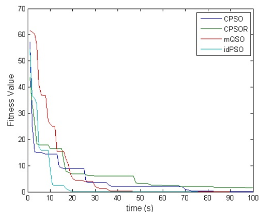
(شکل-۵): مقایسه زمان اجرای الگوریتم‌ها برای مسئله MPB (Figure-5): Comparison of run time algorithms for the MPB problem
