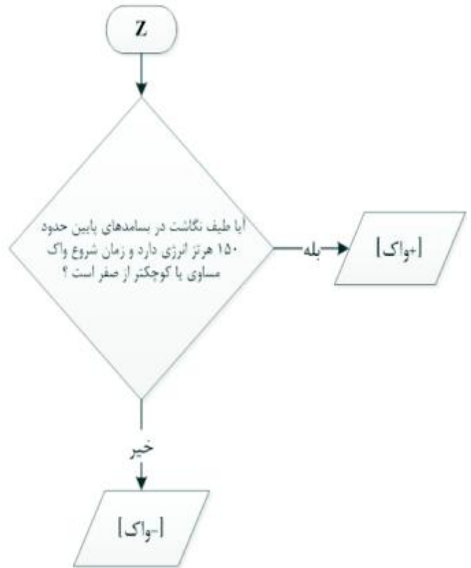
(شکل ۶): نمودار گردش‌ی مربوط به پیمانه Z
