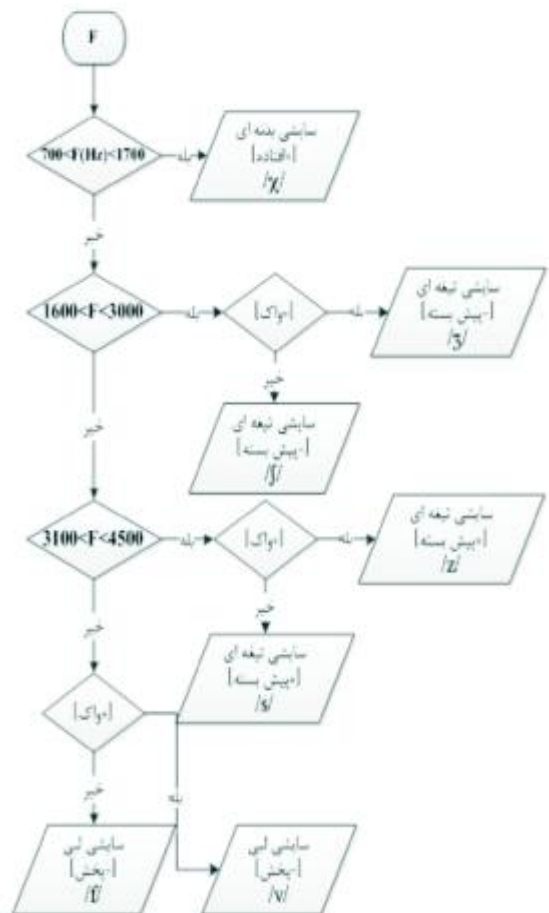
شکل ۱۰): نمودار گردش مربوط به پیمانه F
