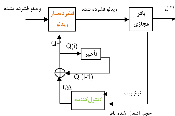
(شکل ۱-۱): نمودار جعبه ای کنترل کننده نرخ بیت ویدئو (Figure-1): Block diagram of the proposed video rate control algorithm
