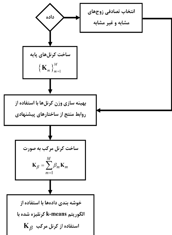
(شکل-۱): نمودار کلی ساختار یادگیری کرنل مرکب در چارچوب یادگیری معیار فاصله (Figure-1): The flowchart of multiple kernel learning method in the distance metric learning framework
