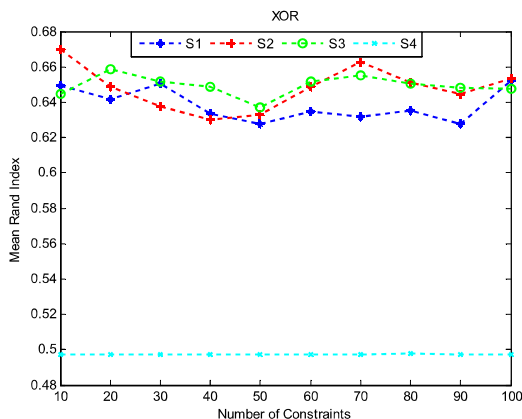
(شکل-۴): متوسط RI روش‌های مختلف بر روی داده XOR. به‌ازای تعداد قیدهای متفاوت. S1 ساختار یک، S2 ساختار دو،
