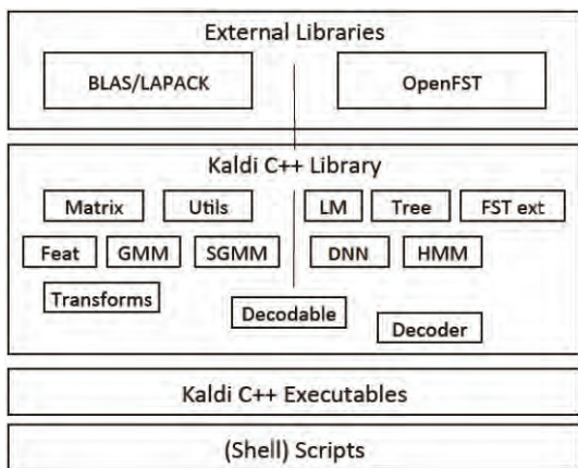
(شکل - ۱): نمایشی ساده‌شده از اجزای نرم‌افزاری سامانه کلدی (Figure-1): A simplified diagram on the software modules from the Kaldi toolkit
