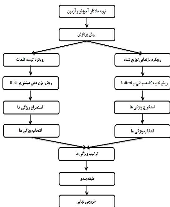
(شکل-۲): چهارچوب مدل پیشنهادی
