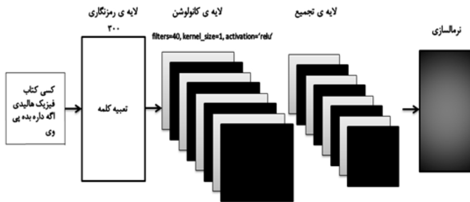
(شکل ۵): معماری مدل دوم پیشنهادی
