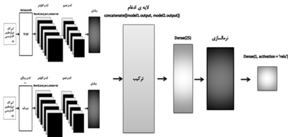
(شکل ۶): معماری مدل پیشنهادی
