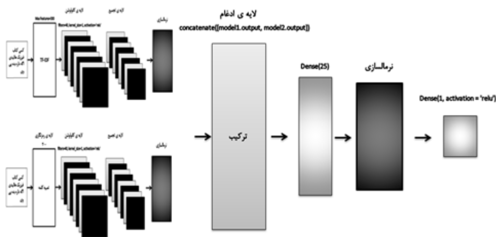
(شکل ۶): معماری مدل پیشنهادی
