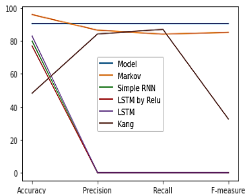
(شکل-۱۰): مقایسه روش پیشنهادی با روش‌های پیشین
