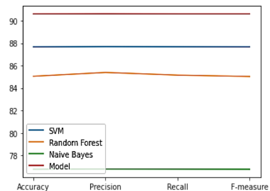
(شکل-۹): مقایسه روش پیشنهادی با روش‌های مبتنی بر
