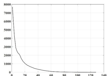
(شکل-۴): نتایج الگوریتم PCA با ۱۲۸ ویژگی (Figure-4): PCA Result for the 128 features
